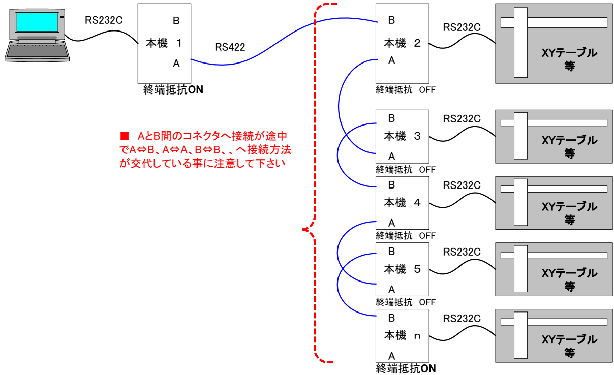
1:n接続例
