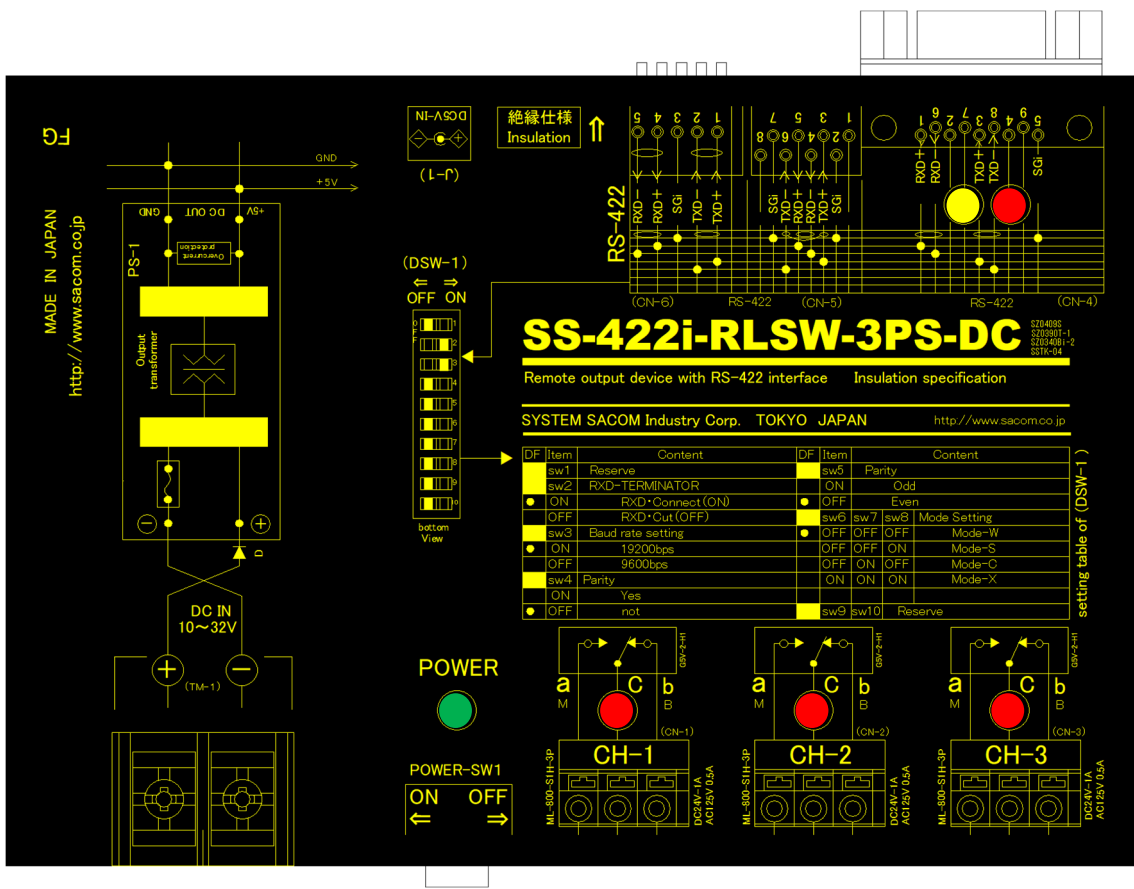
上図はSS-422i-RLSW-3PS-DC
