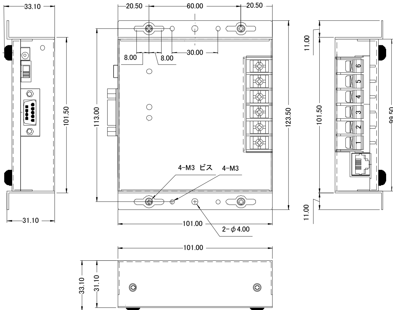
寸法図
