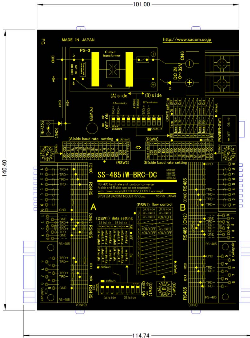
本体寸法図
