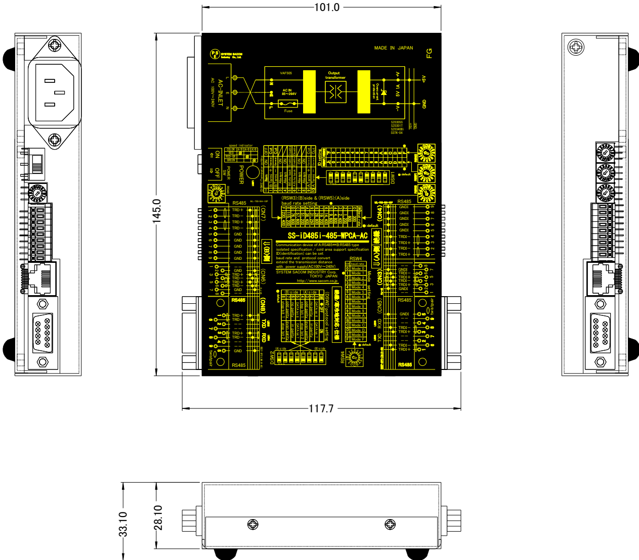
本体寸法図
