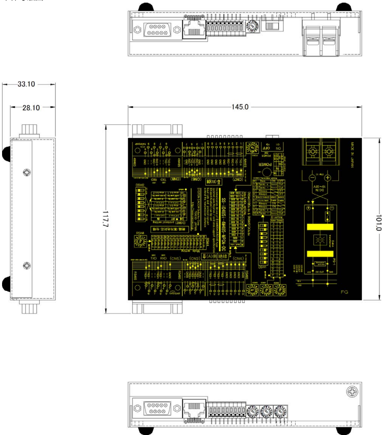
本体寸法図
