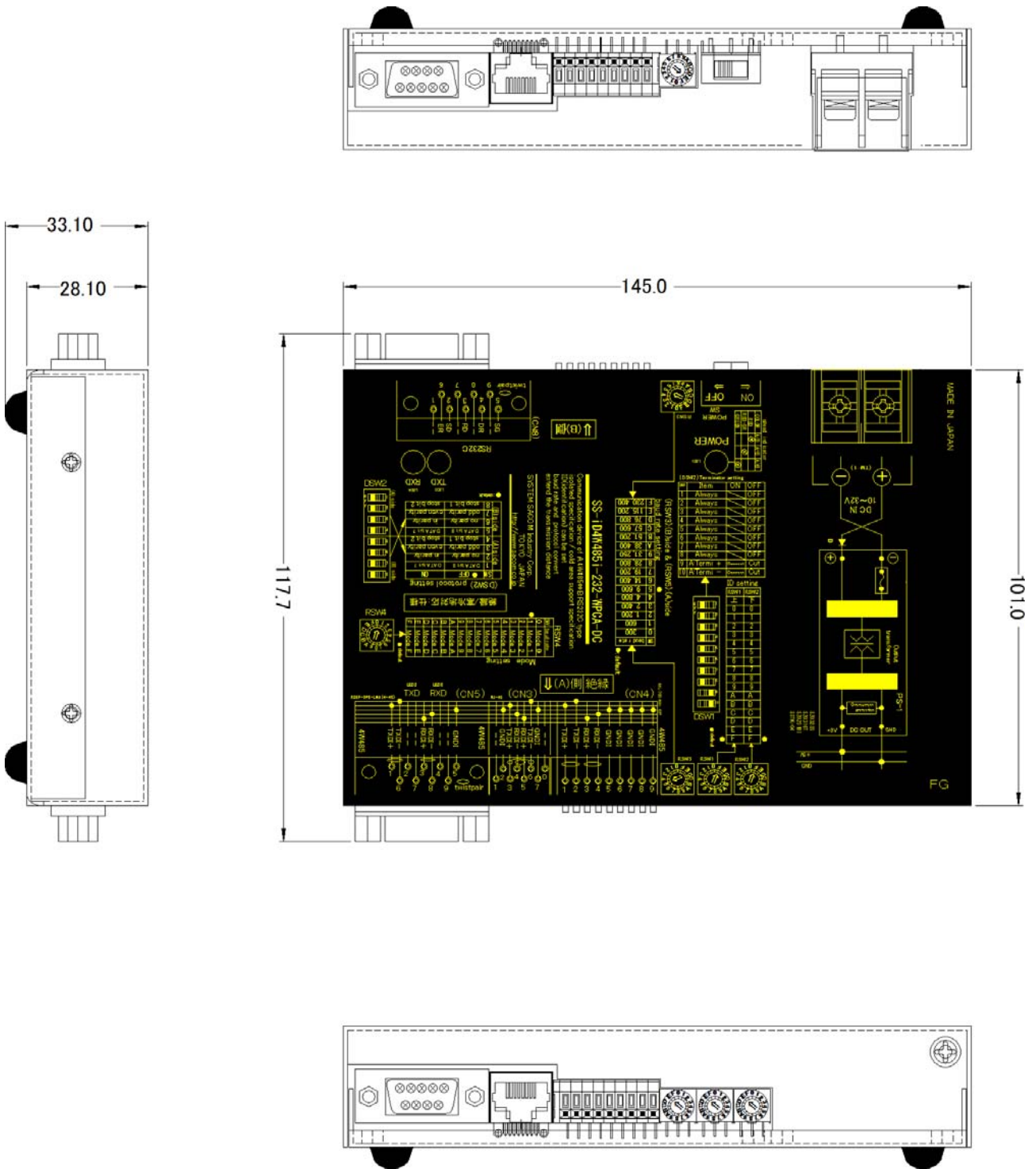
本体寸法図
