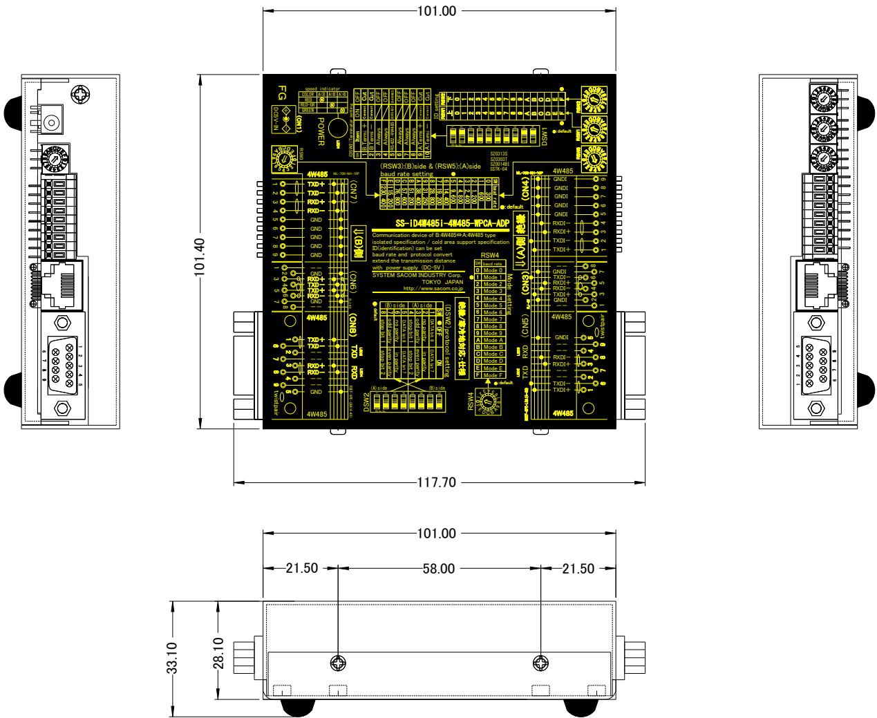
本体寸法図
