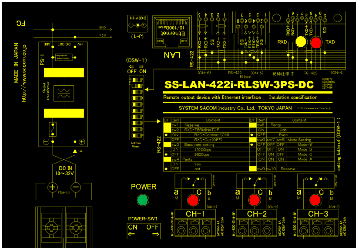
上図はSS-LAN-422i-RLSW-3PS-DC
