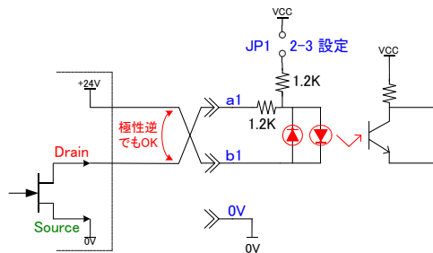
絶縁：オープンドレイン
