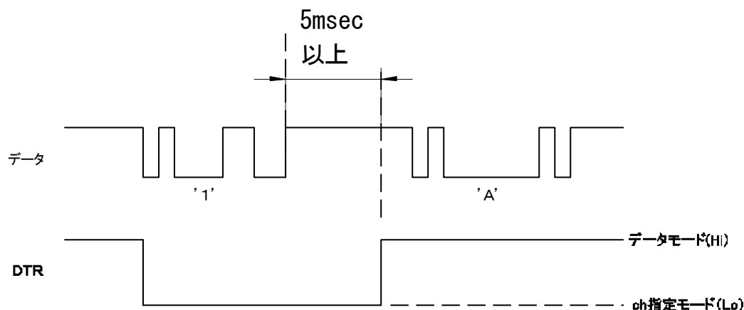
(例)コモン CH とサブ CH-1 と回線を開いてデータ 'A' を送るタイミングチャート
