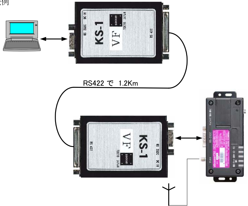
接続例
