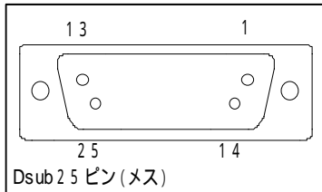
KS-232SP/KS-232PS のシリアル側 (共通配列)
