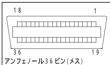
KS-232SPの平行側
